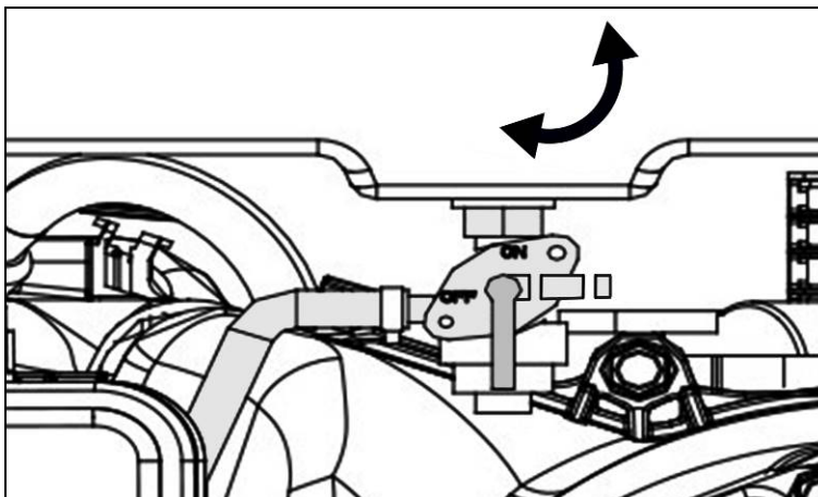
Рис. 8. Топливный кран
