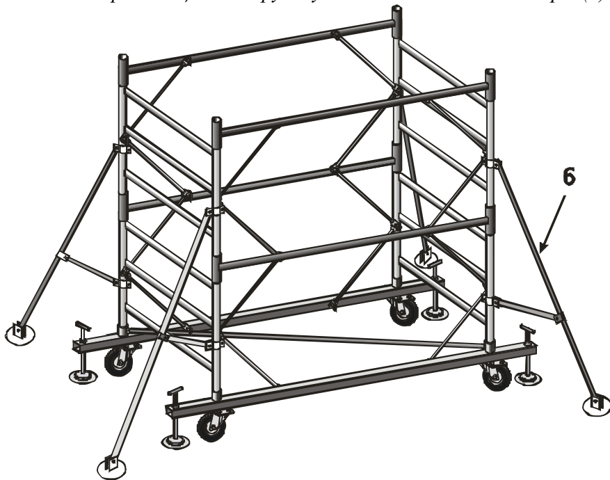
6.6. Собрать вышку на требуемую высоту, установив объемные диагонали в каждом четвертом ярусе. Завершается вышка секцией ограждения, сборка которой описана ниже.
