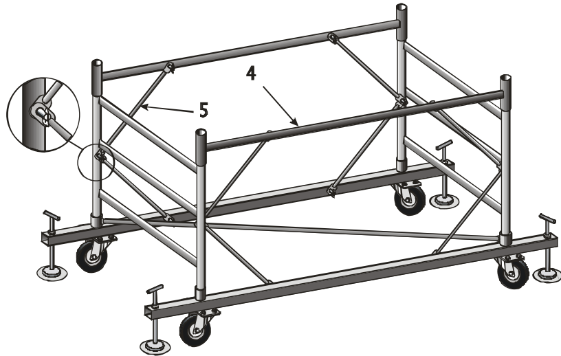
6.5. Собрать еще один ярус и установить стабилизаторы (6).
