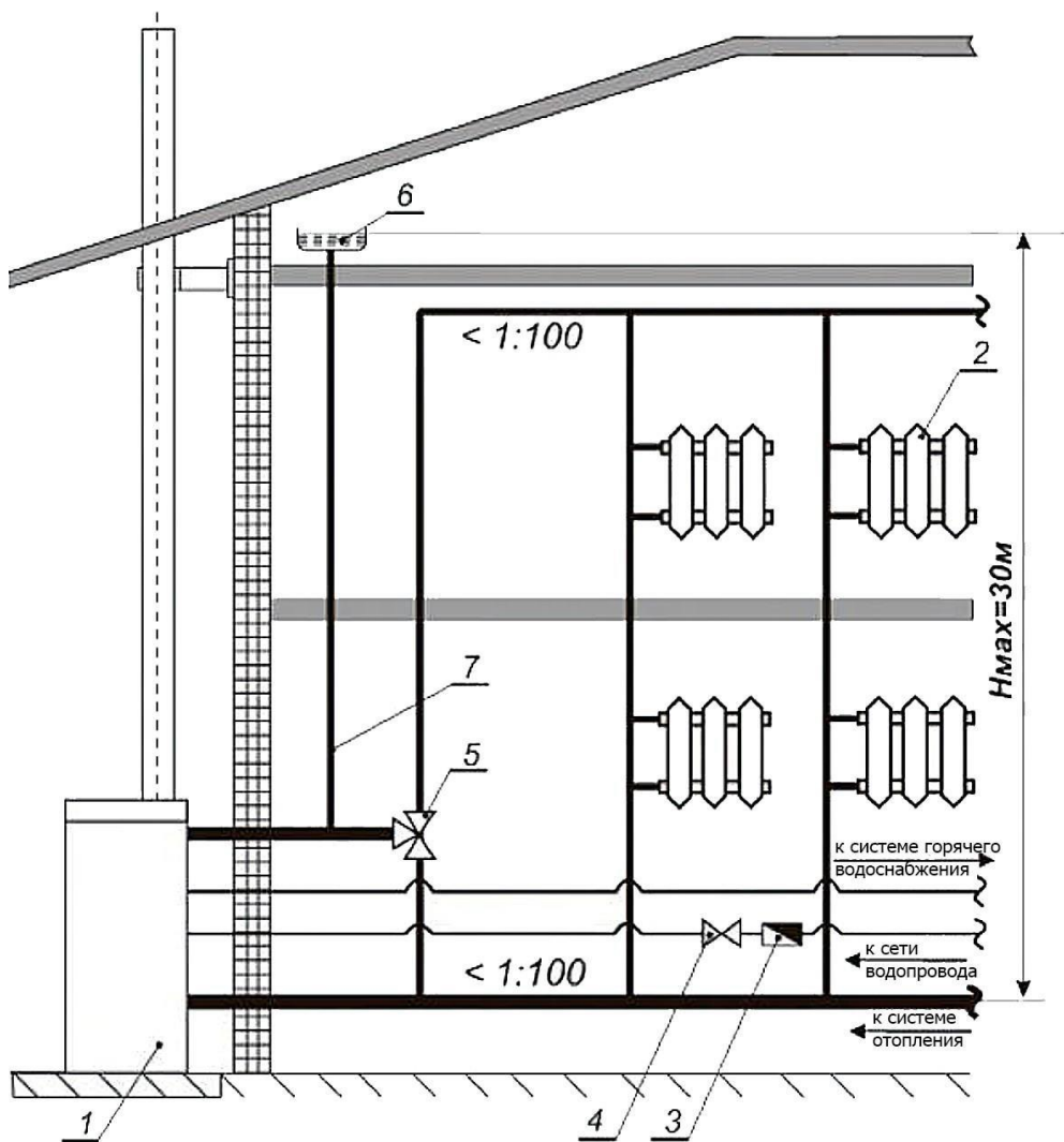
Рис. 2а Схема монтажа котла, системы отопления и горячей водоснабжения с естественной циркуляцией теплоносителя в котле (рекомендуемая)
