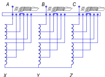
Схема соединения обмоток "ЗВЕЗДА"
