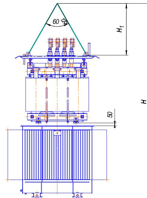
Схема строповки активной части с крышкой при сборке и разборке трансформатора.
