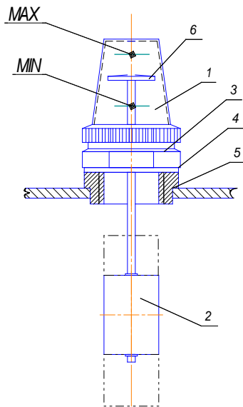
Рисунок 9 – Маслоуказатель
