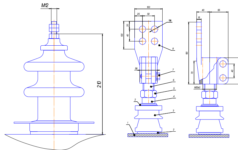
Рисунок 5 - ввод ВН
