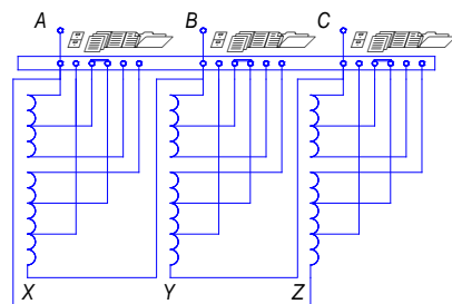
Схема соединения обмоток "ТРЕУГОЛЬНИК"
