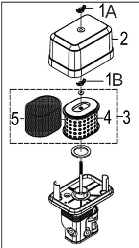
Рис. 15 Обслуживание воздушного фильтра
