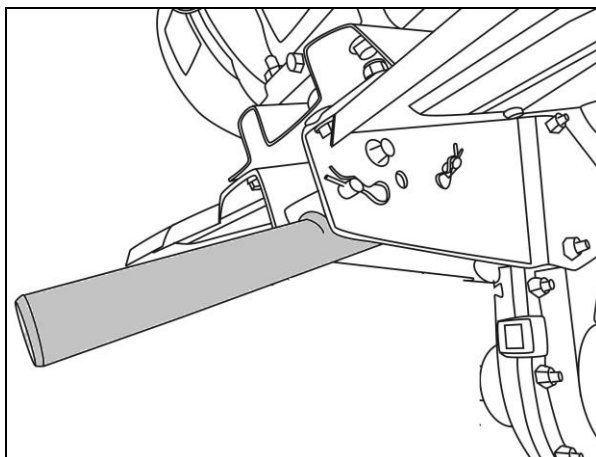
Рис. 9. Кронштейн
