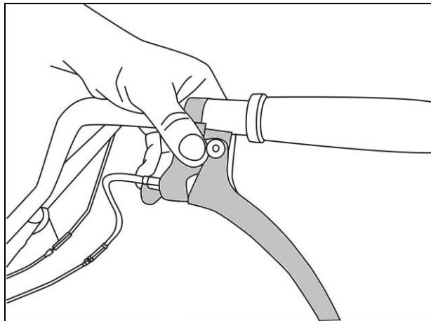
Рис. 6. Установка рукоятки
