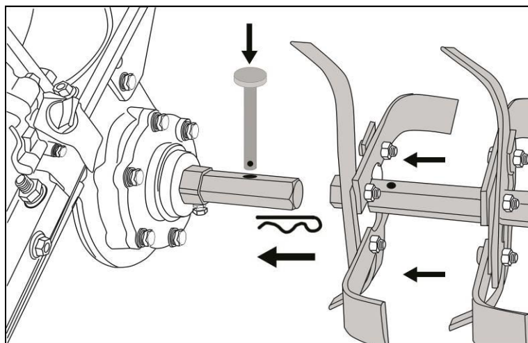
Рис. 8. Установка фрезы
