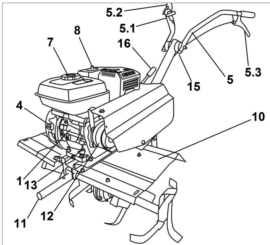
Рис. 1. Общий вид 1
