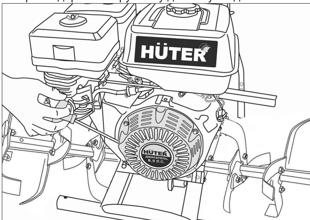
Рис. 25. Запуск двигателя ручкой стартера
