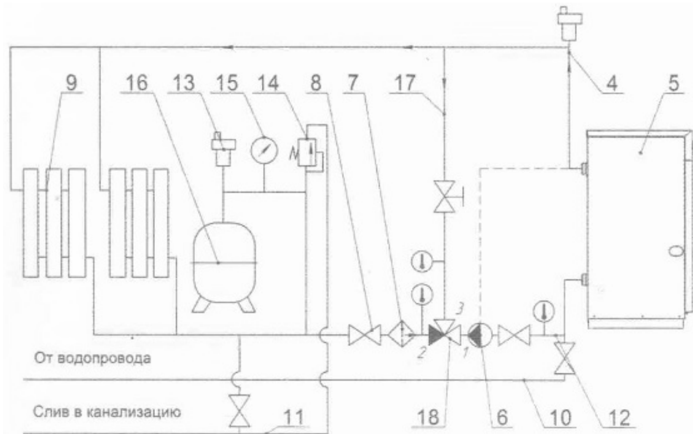
Рис.6. Рекомендуемая гидравлическая закрытая схема системы отопления с байпасной линией рециркуляции, автоматическим трехходовым клапаном для прогрева теплоносителя в теплообменнике котла в целях исключения образования конденсата.
