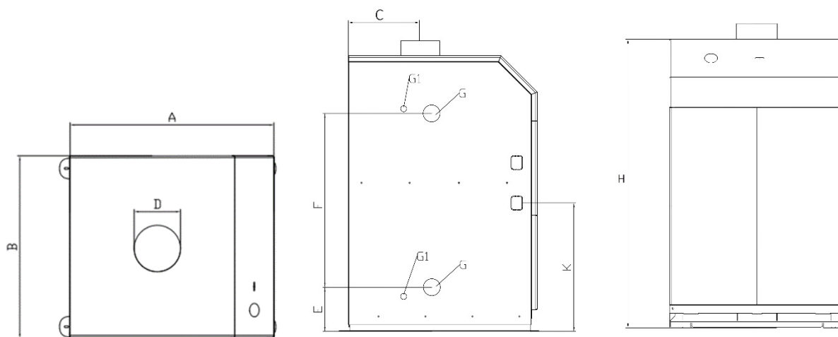
Рис.2 Общий вид и размеры КОГВ «STRATTOS» 70-100 кВт
