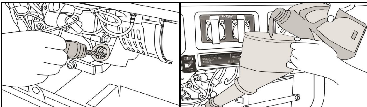
Рис. 8. Заправка маслом
