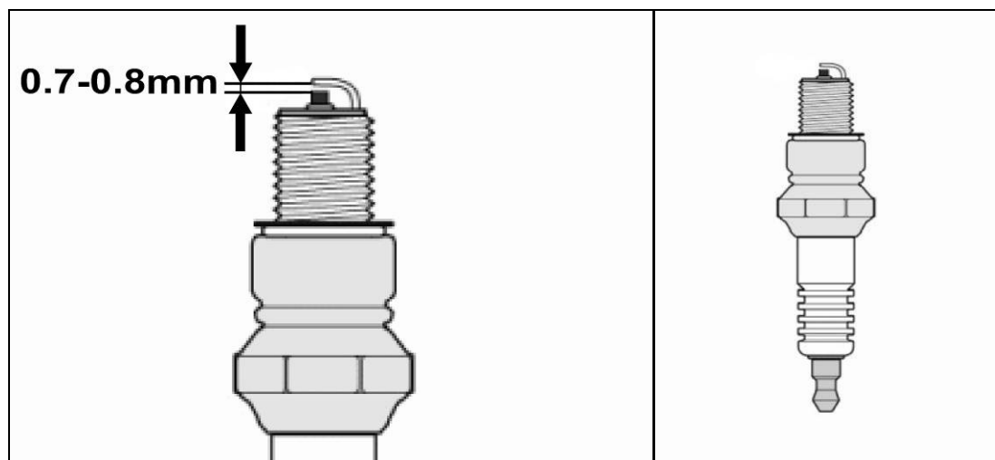
Рис. 25. Свеча зажигания
