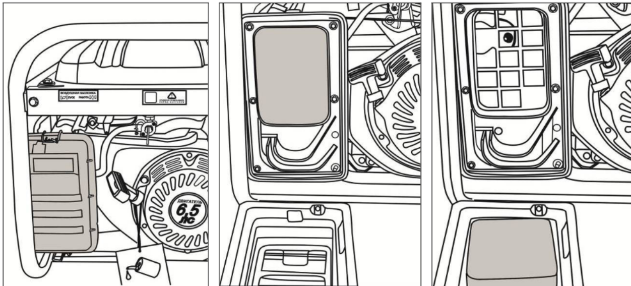
Рис. 26. Воздушный фильтр
