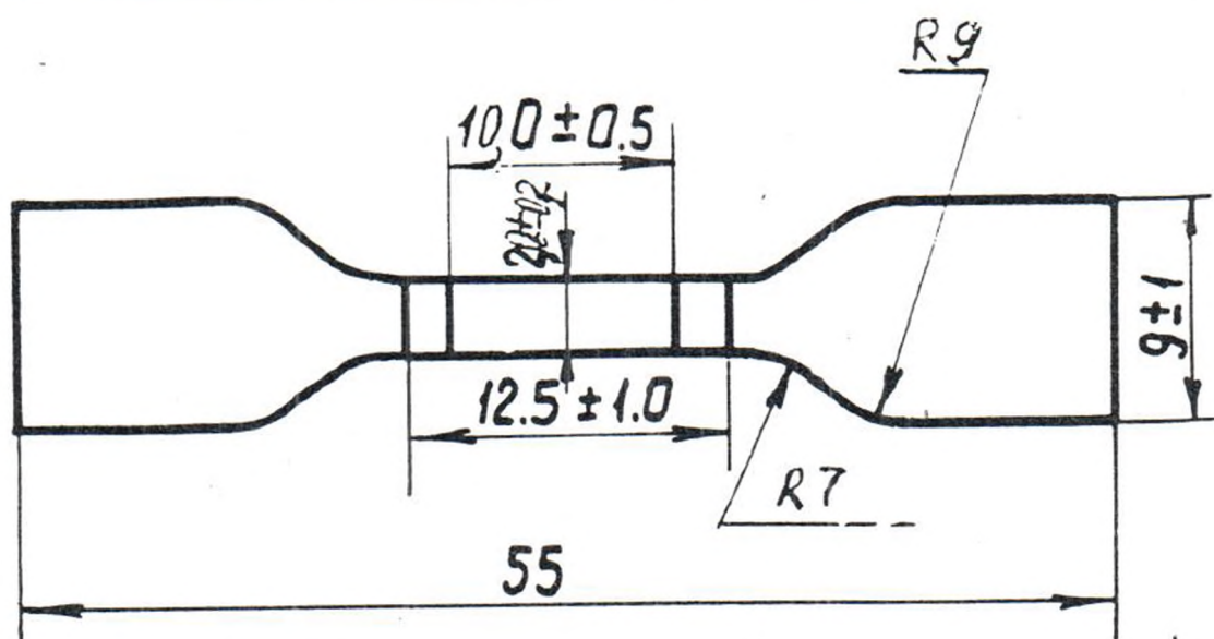
Рисунок 1 - Лопатка
